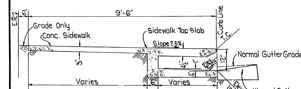
SECTION G-G FROM STA. 100+02 TO STA. 100+08
