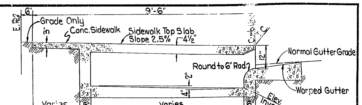
SECTION A-A FROM STA. 98+04 TO STA. 98+18
